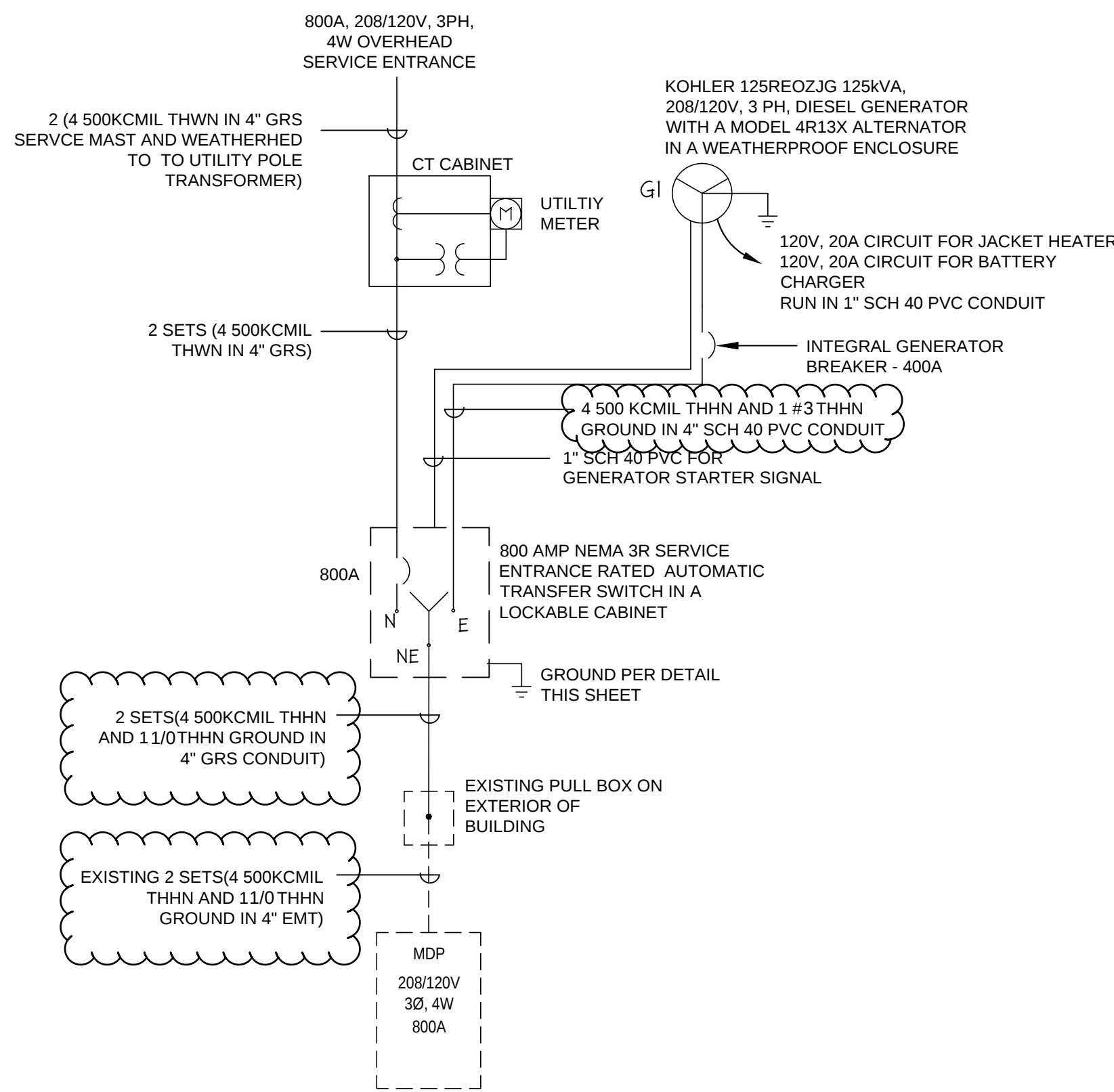
2 SINGLE LINE DIAGRAM E1 SCALE: N.T.S.
