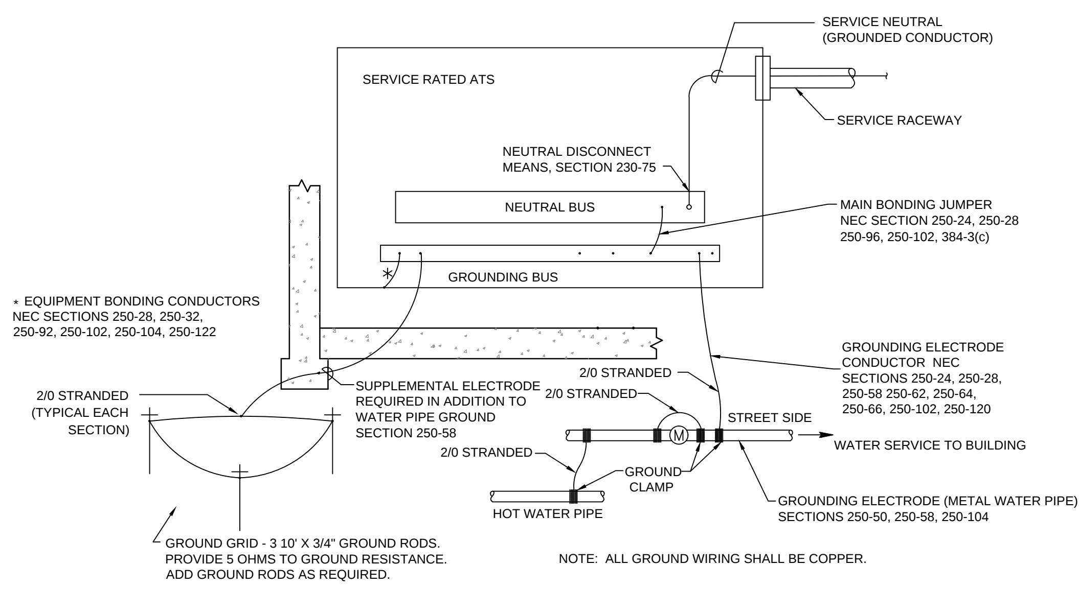
3 SERVICE GROUNDING DETAIL E1 SCALE: N.T.S.
